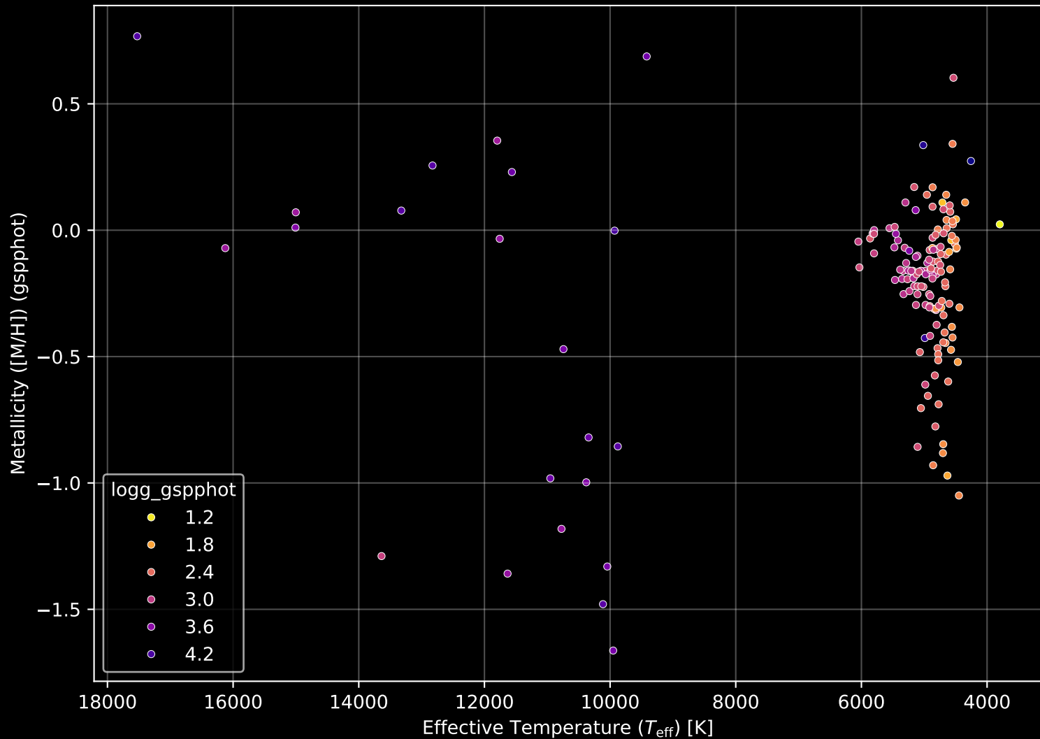
APOGEE DR17 Field: [225+04] Stellar Population Parameters (n= 164)
